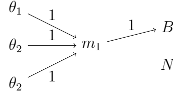
(d) PBE and BPE for 9c
