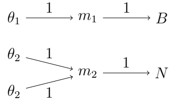
(b) PBE and BPE for 9a
